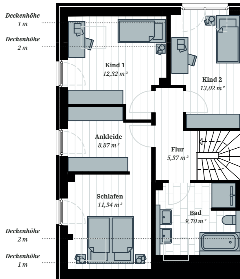
DACHGESCHOSS
